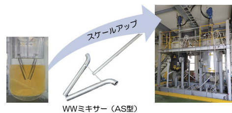
WWミキサー (AS型)
